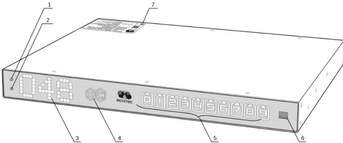
Рисунок 4.1.3. Лицевая панель RPCM DC 232A.
