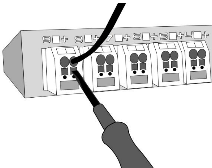
Рисунок 2.2.7. Подключение проводника к клемме вывода RPCM DC ATS 76A или RPCM DC 232A.
