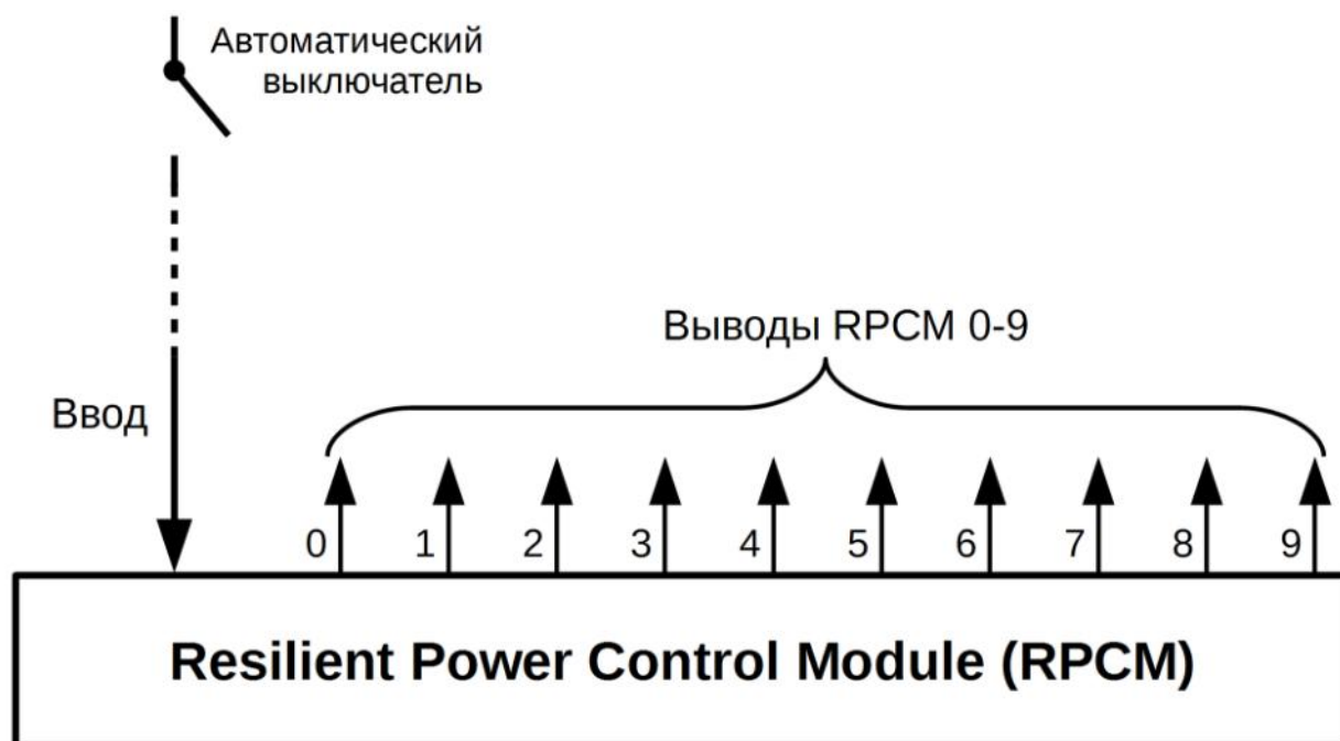
Рисунок 2.2.4. Схема подключения RPCM DC 232A.
