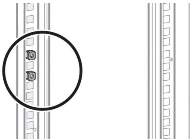
Рисунок 2.2.1. Установка клетевых стоечных гаек в монтажной стойке.
