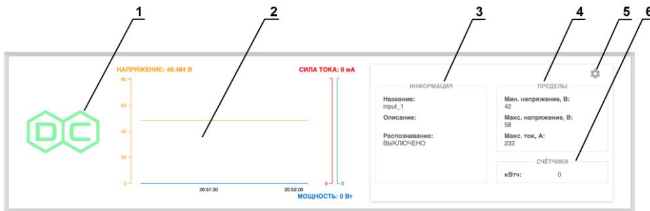
Рисунок 4.4.8. Информационная область ввода RPCM DC ATS 76A.
