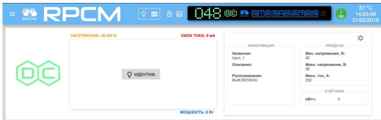
Рисунок 4.4.9. Область управления вводом в режиме Control Mode для RPCM DC 232A.
