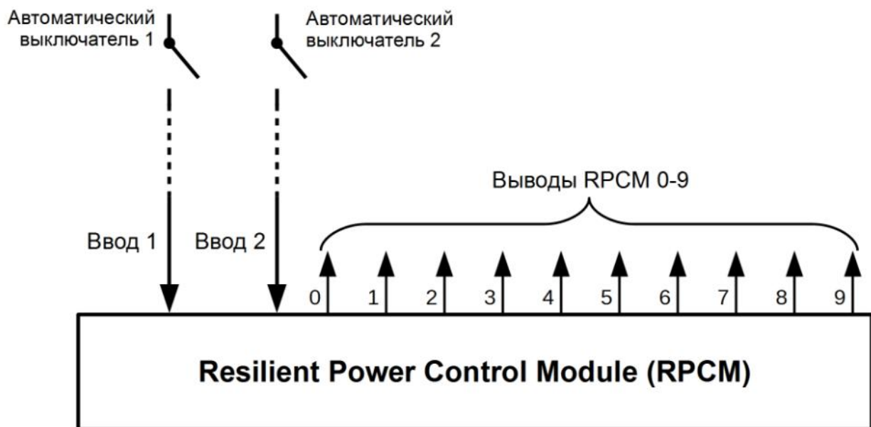
Рисунок 2.2.3. Схема подключения RPCM DC ATS 76A.
