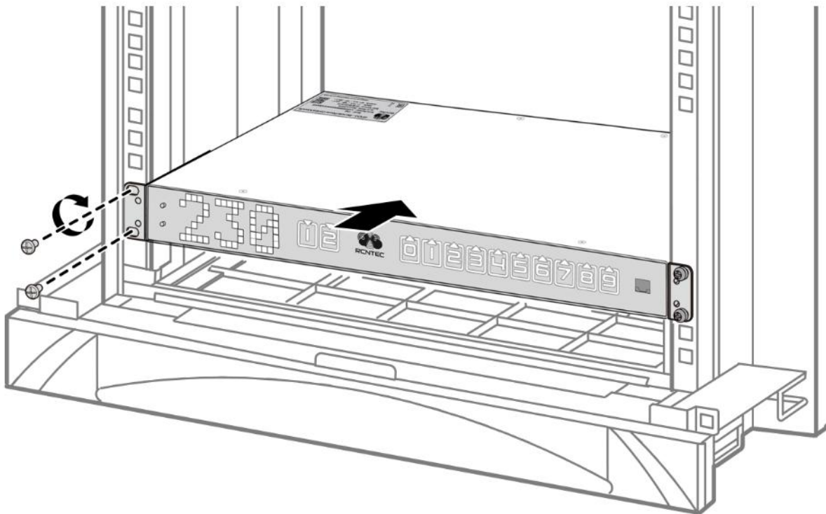
Рисунок 2.2.2. Установка модуля RPCM.
