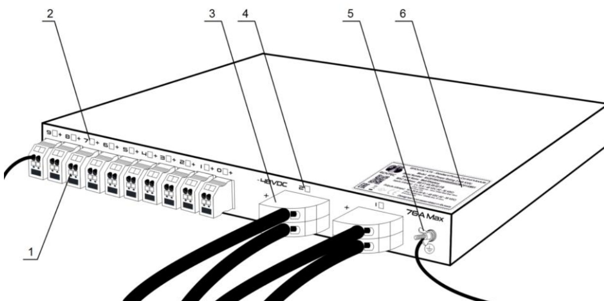
Рисунок 4.1.2. Задняя сторона RPCM DC ATS 76A.
