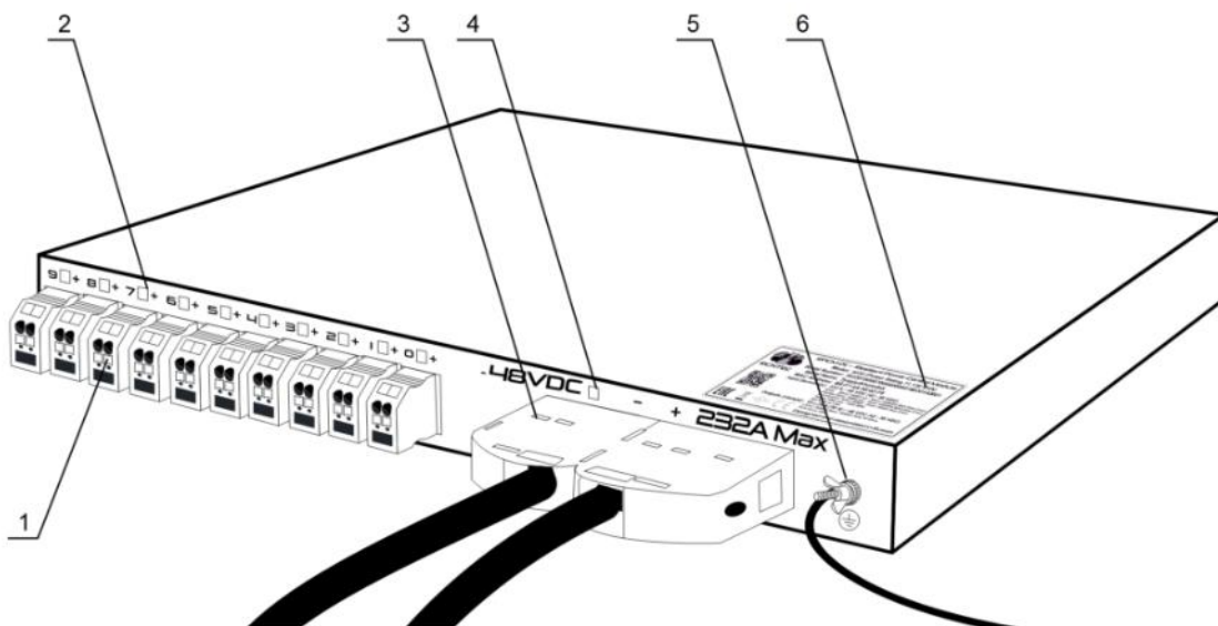
Рисунок 4.1.4. Задняя сторона RPCM DC 232A.
