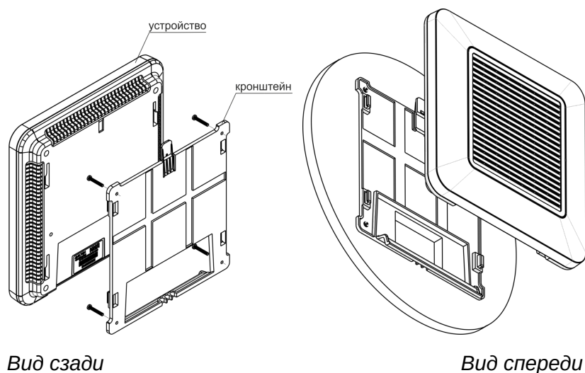
Рисунок 8 – Установка устройства
