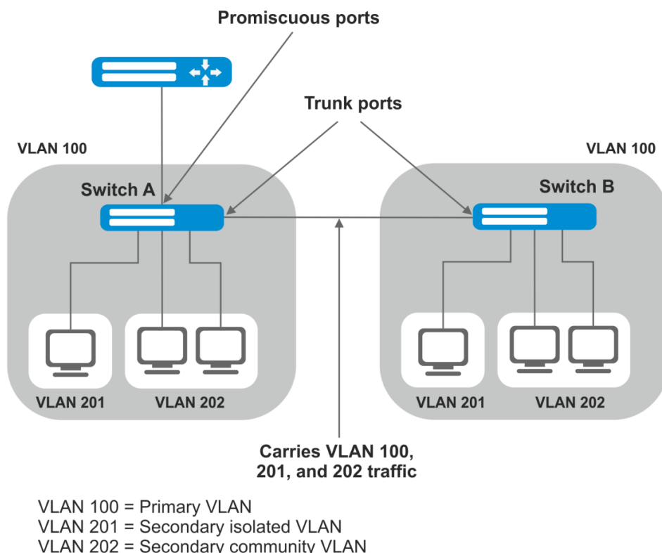
Рисунок 46 – Пример работы технологии Private VLAN
