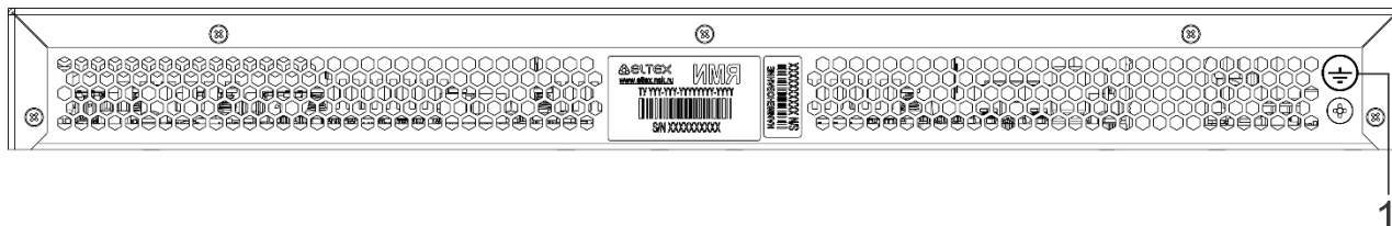
Рисунок 11 – Задняя панель MES2300-24
