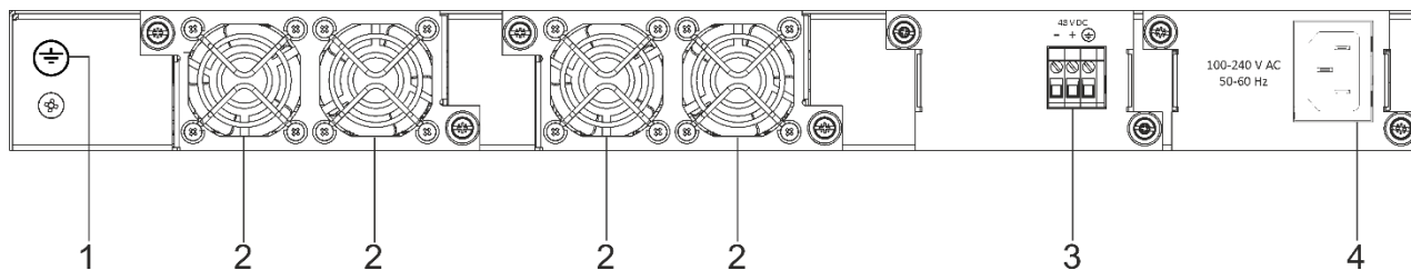
Рисунок 16 – Задняя панель MES5400-24
