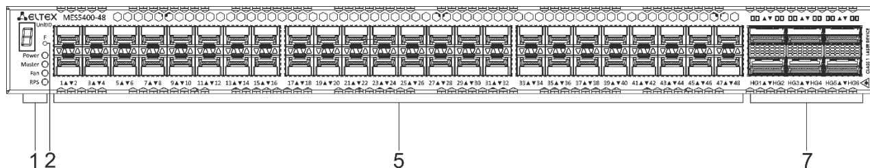
Рисунок 9 – Передняя панель MES5400-48
