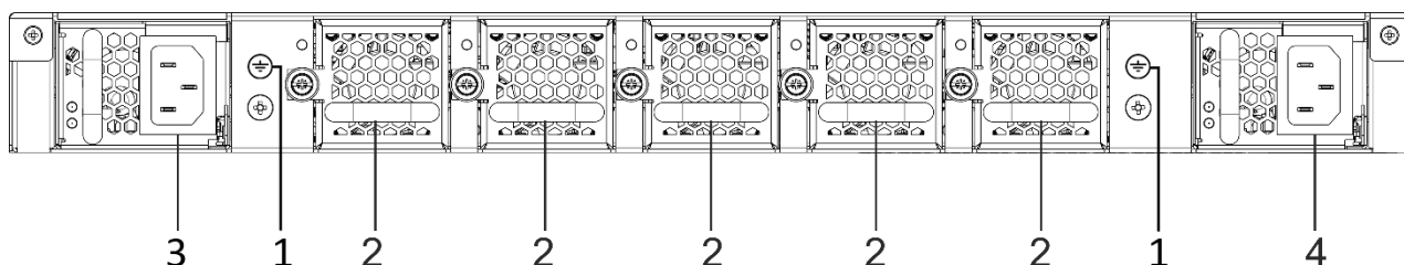
Рисунок 18 – Задняя панель MES5500-32
