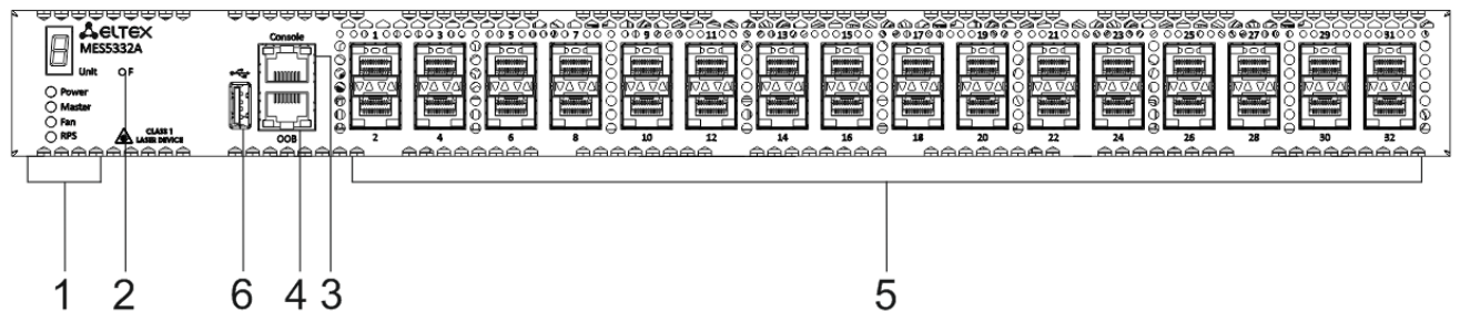
Рисунок 7 – Передняя панель MES5332A
