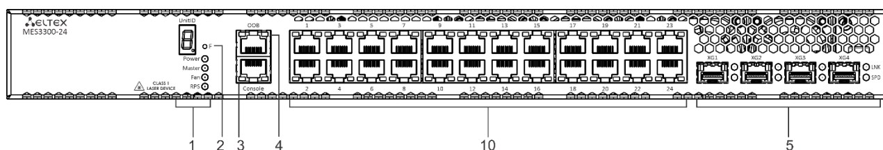
Рисунок 2 – Передняя панель MES3300-24
