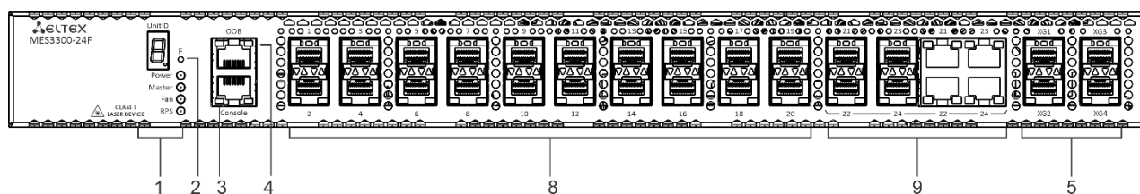
Рисунок 3 – Передняя панель MES3300-24F
