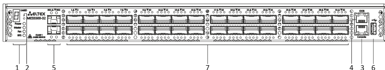
Рисунок 10 – Передняя панель MES5500-32
