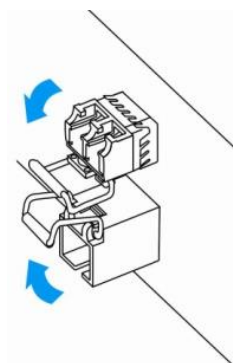
Рисунок 44 – Открытие защелки SFP-трансиверов
