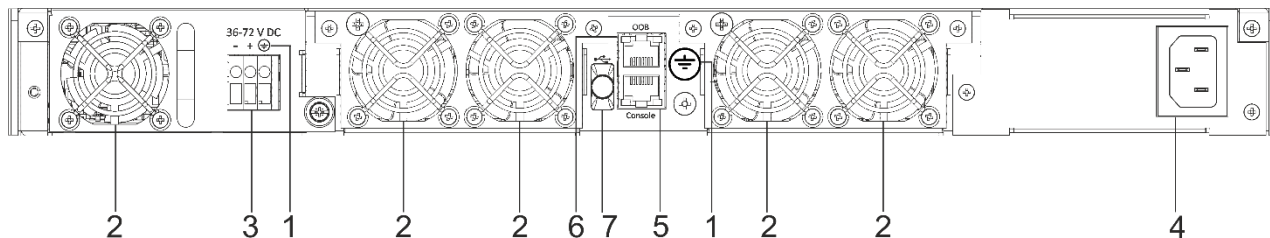
Рисунок 17 – Задняя панель MES5400-48
