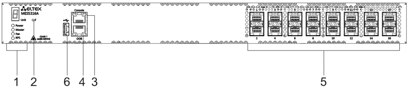
Рисунок 5 – Передняя панель MES5316A
