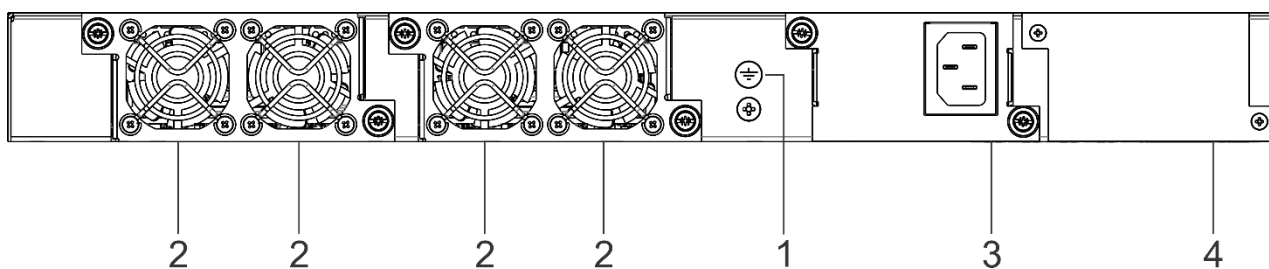
Рисунок 13 – Задняя панель MES3300-24F
