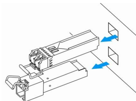
Рисунок 45 – Извлечение SFP-трансиверов
