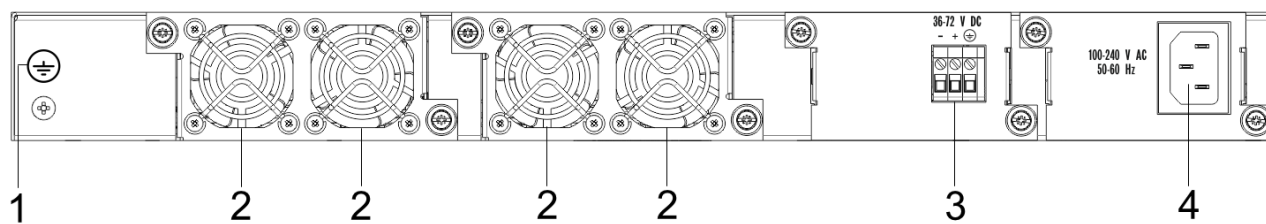
Рисунок 14 – Задняя панель MES5312, MES5324A, MES5332A
