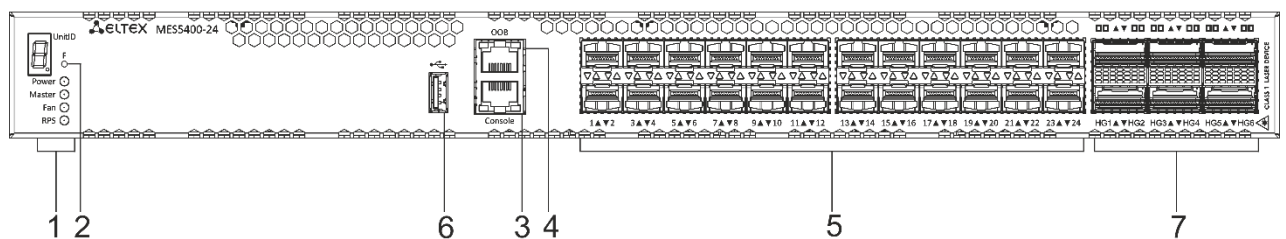
Рисунок 8 – Передняя панель MES5400-24
