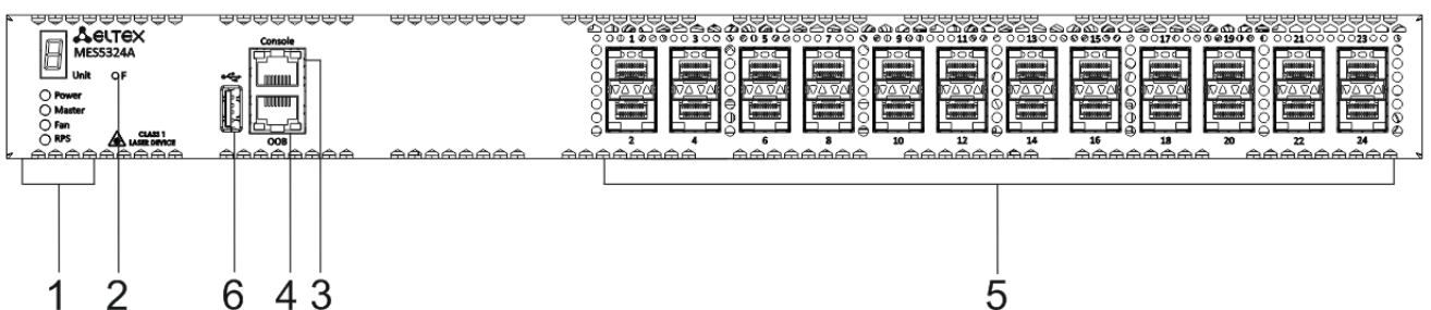
Рисунок 6 – Передняя панель MES5324A Внешний вид передней панели устройств MES5332A показан на рисунке 7.
