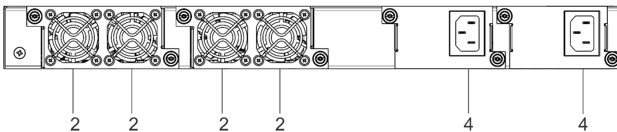
Рисунок 12 – Задняя панель MES3300-24
