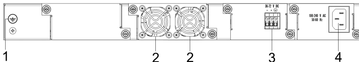
Рисунок 15 – Задняя панель MES5316A
