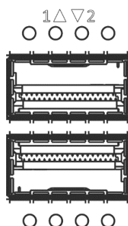
Рисунок 34 – Внешний вид разъема QSFP+ и QSFP28 для MES5500-32
