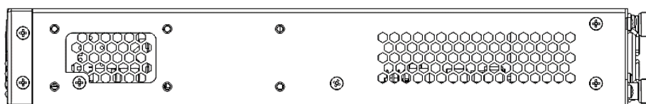
Рисунок 23 – Правая боковая панель MES5316A, MES5324A, MES5332A
