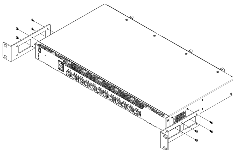
Рисунок 36 – Вариант крепления кронштейнов №2
