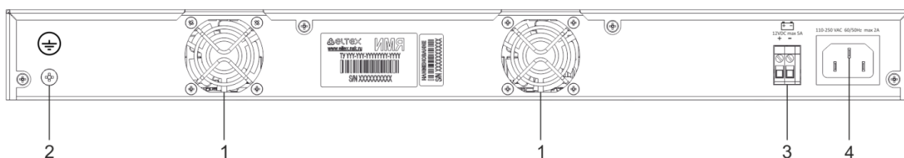
Рисунок 28 – Задняя панель MES2448B
