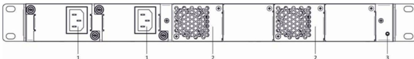
Рисунок 14 – Внешний вид задней панели SMG-1016M
