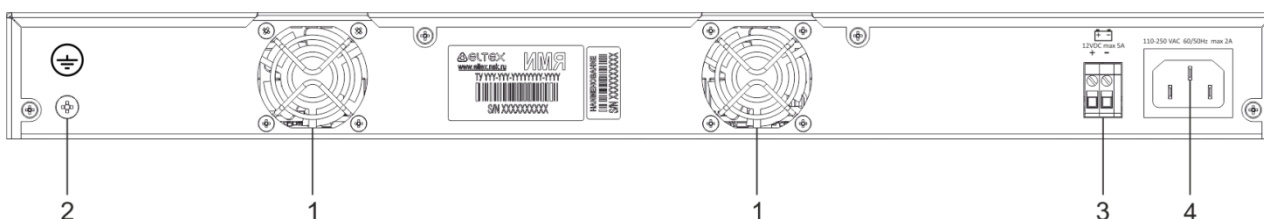
Рисунок 27 – Задняя панель MES2448B
