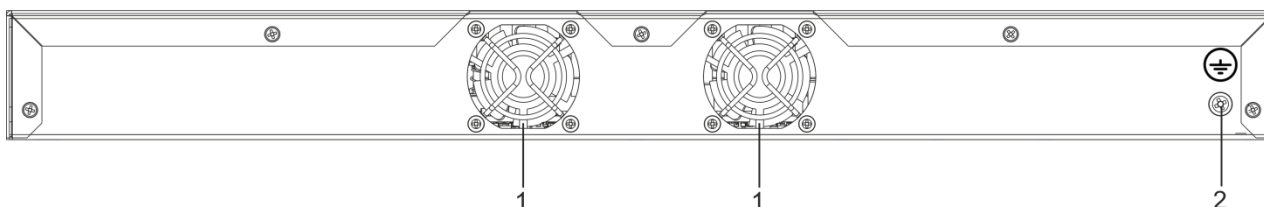
Рисунок 25 – Задняя панель MES2428P
