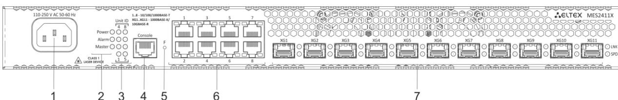
Рисунок 22 – Передняя панель MES2411X
