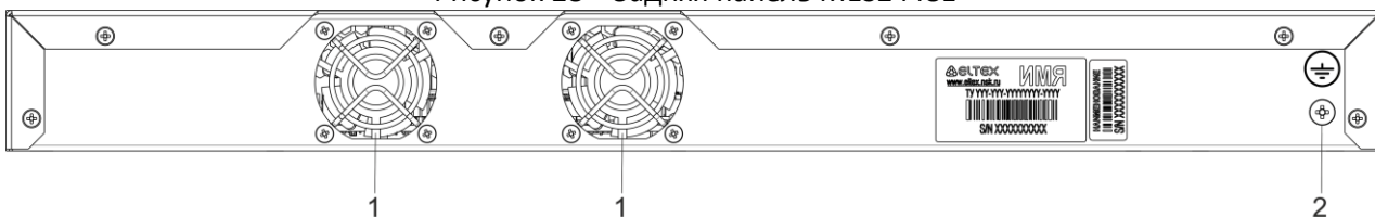
Рисунок 29 – Задняя панель MES2411X
