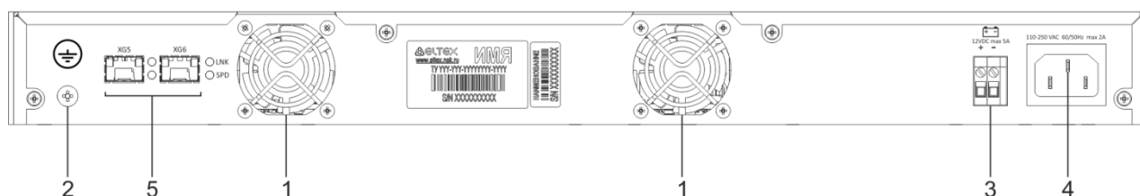
Рисунок 28 – Задняя панель MES2448E
