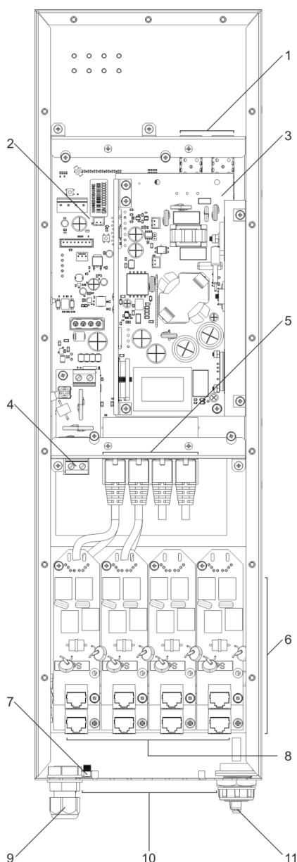
Рисунок 32 – Основные компоненты и разъемы MES3708P
