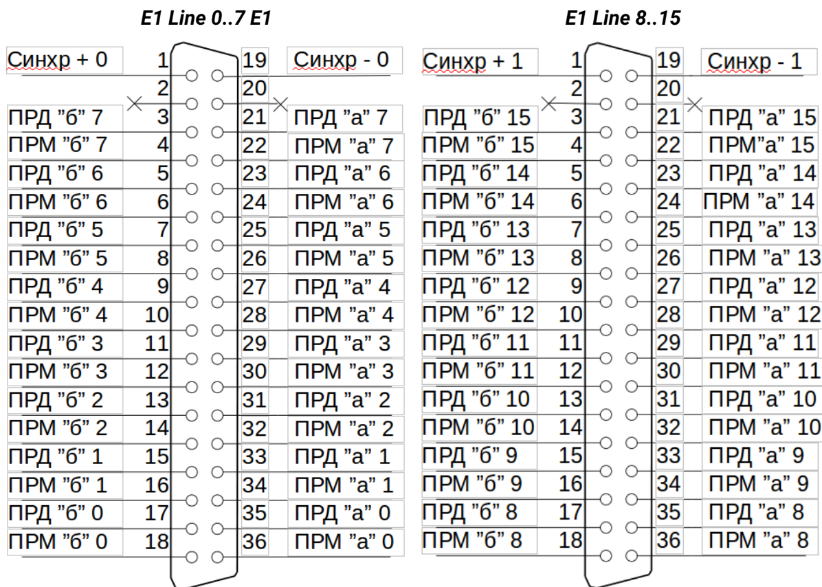
Рисунок 31 – Назначение контактов разъемов E1 Line
